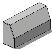
BORDILLO C3 100x28x17-14 / 50x28x17-14 cm
