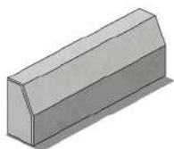
BORDILLO A2 100x20x10-9 / 50x20x10-9 cm
