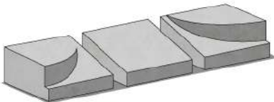
BORDILLO VADO 40x40x18-7 cm
