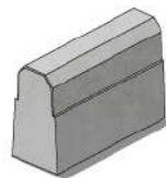
BORDILLO 50x40x22x18-12 cm
